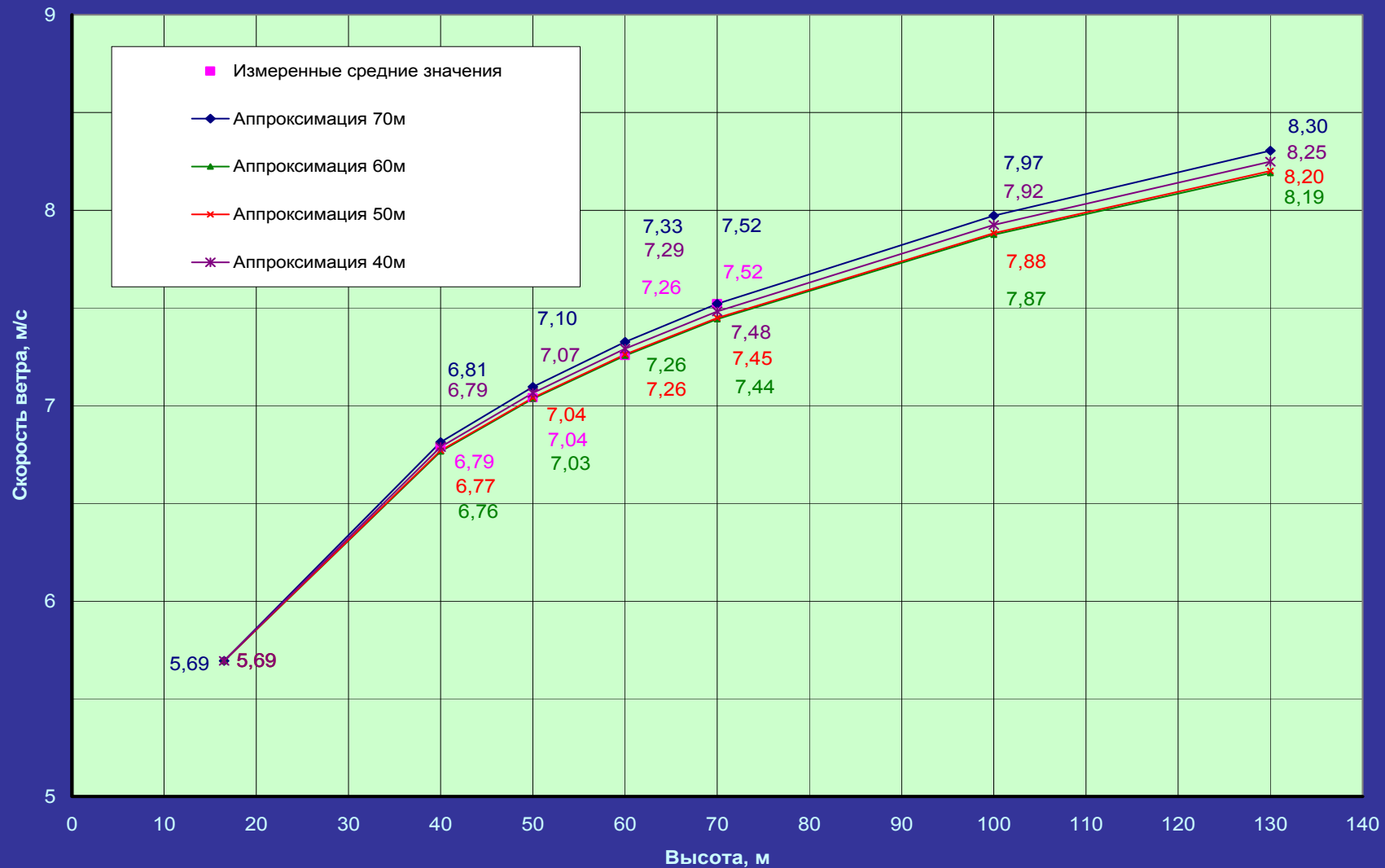
Сравнение средних измеренных и расчетных по логарифмической зависимости высотных профилей скорости ветра для п.Симоновка. Март 2008
